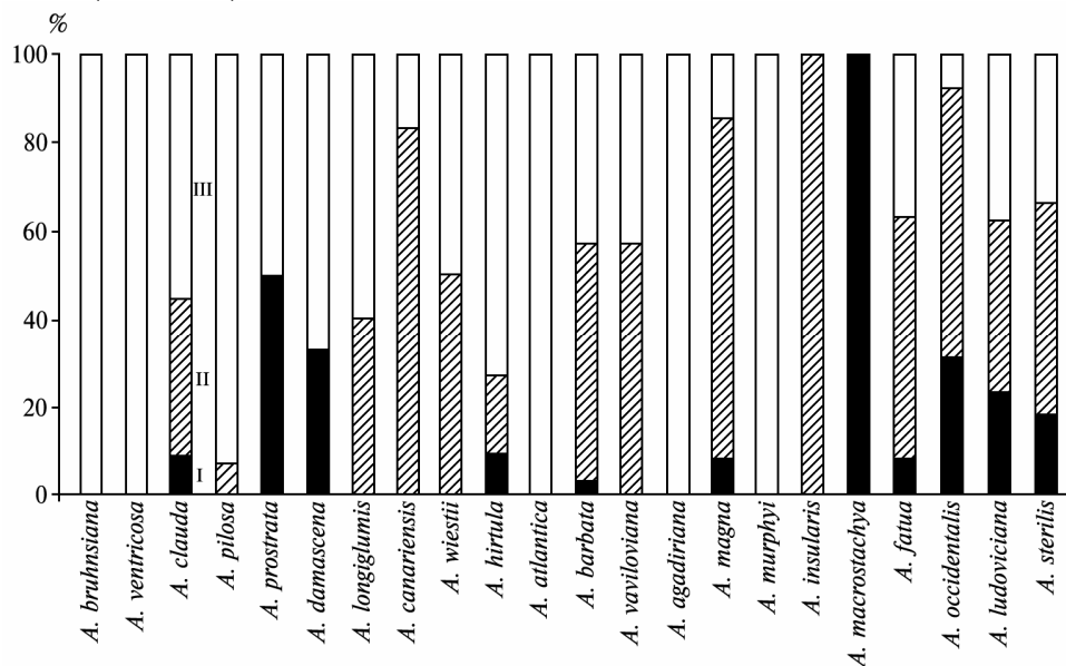
Характеристика дикорастущих видов овса из коллекции ВИР по степени толерантности к вирусу желтой карликовости ячменя (Ленинградская обл., г. Пушкин, 1988-2002 годы): I, II и III — толерантность соответственно 0-1, 3-5 и 7-9 баллов.
